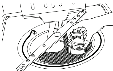
Para quitar el ensamblaje del filtro superior
